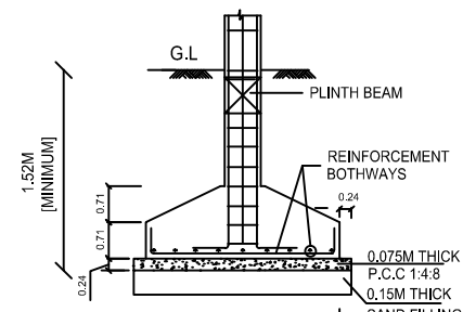
TYP. DET. COLUMN FOOTING
