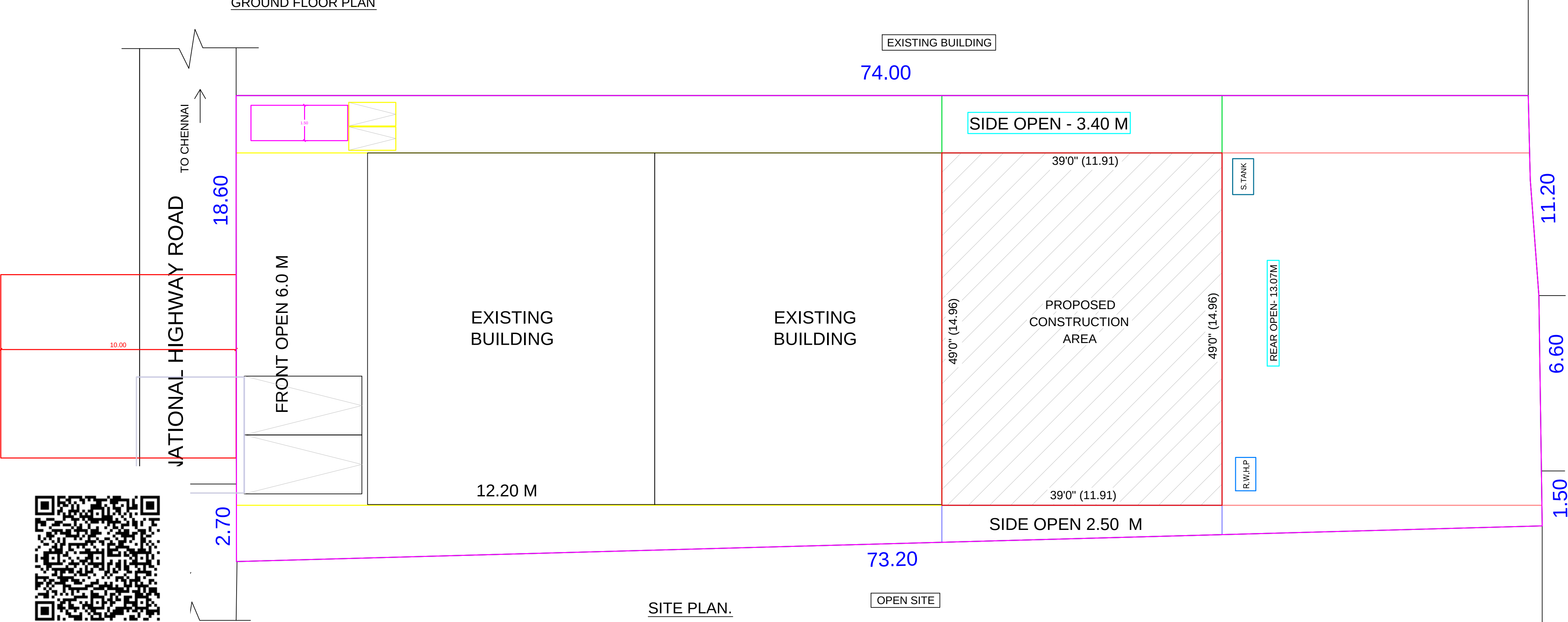
SITE PLAN.
