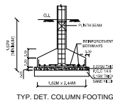
TYP. DET. COLUMN FOOTING
