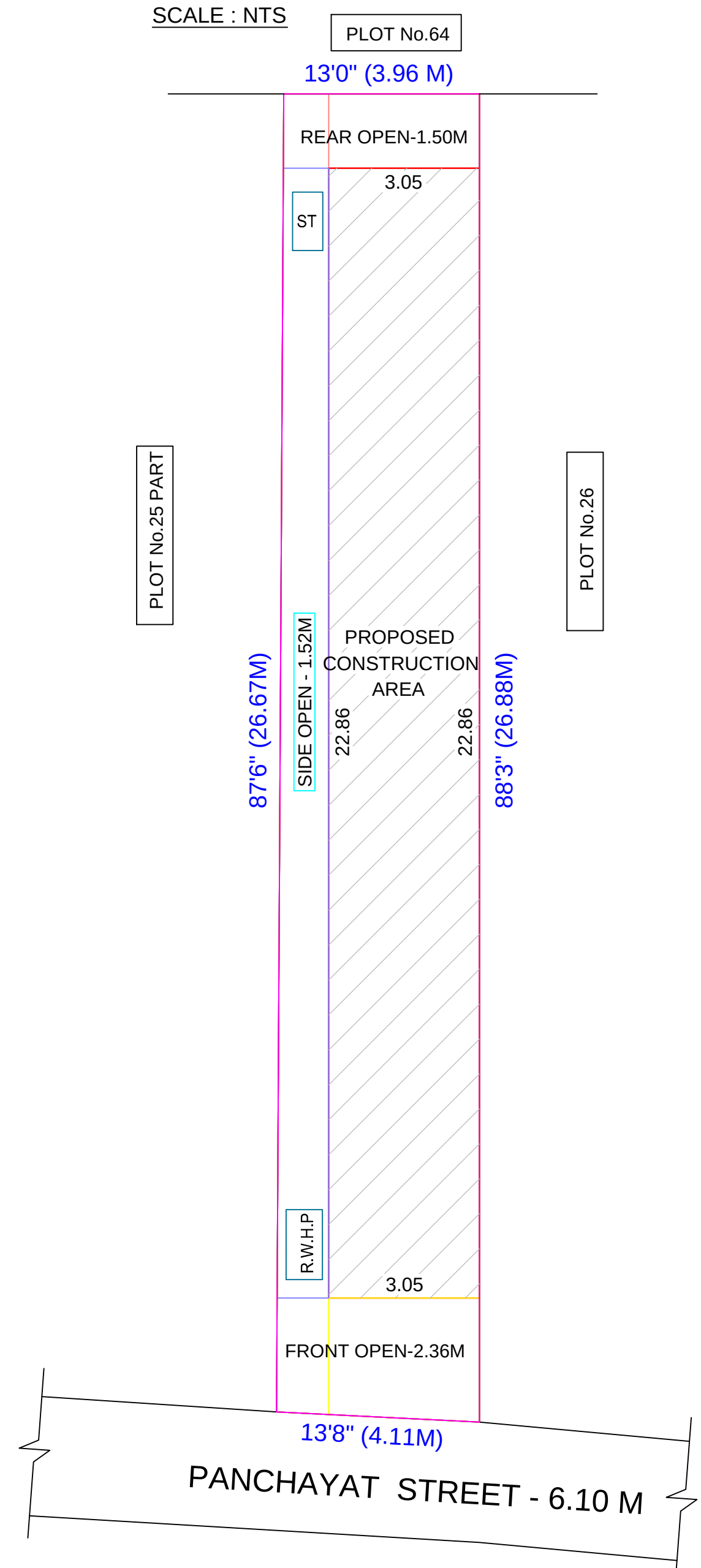
SITE PLAN.
