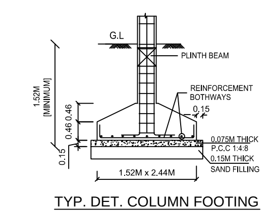
TYP. DET. COLUMN FOOTING
