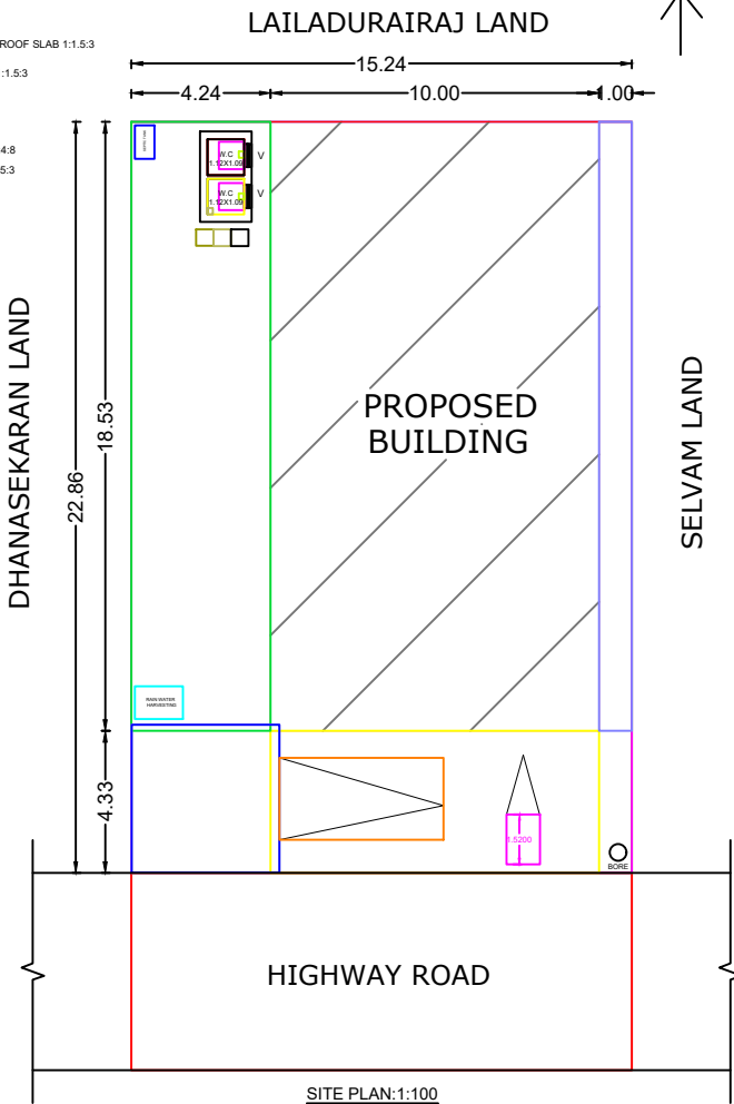
SITE PLAN: 1:100
