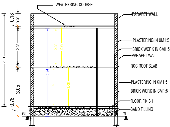
SECTION - EF'
