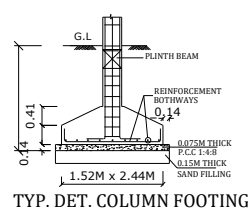
TYP. DET. COLUMN FOOTING
