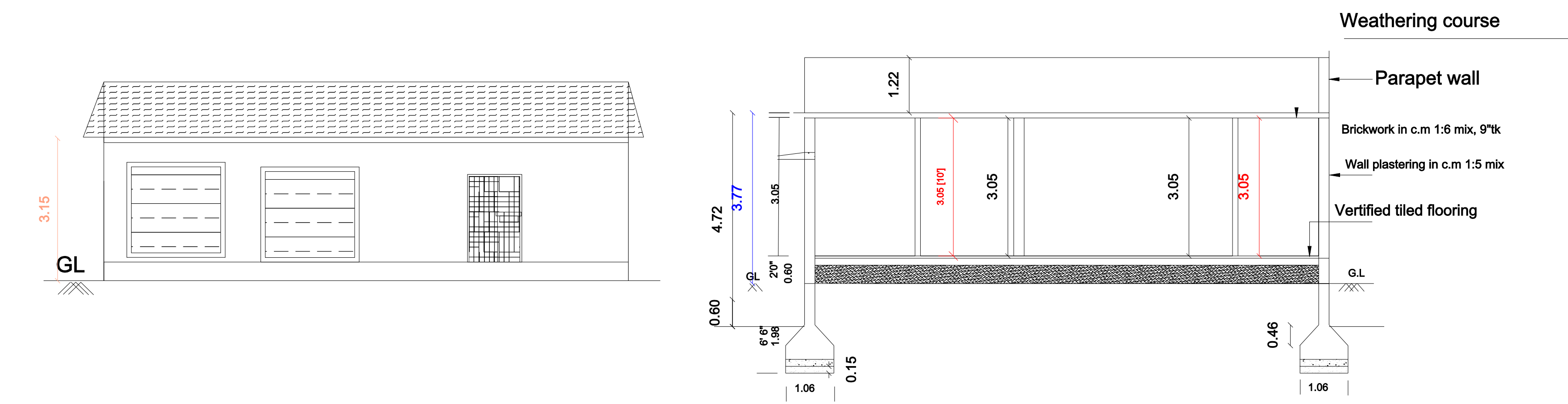
ELEVATION
