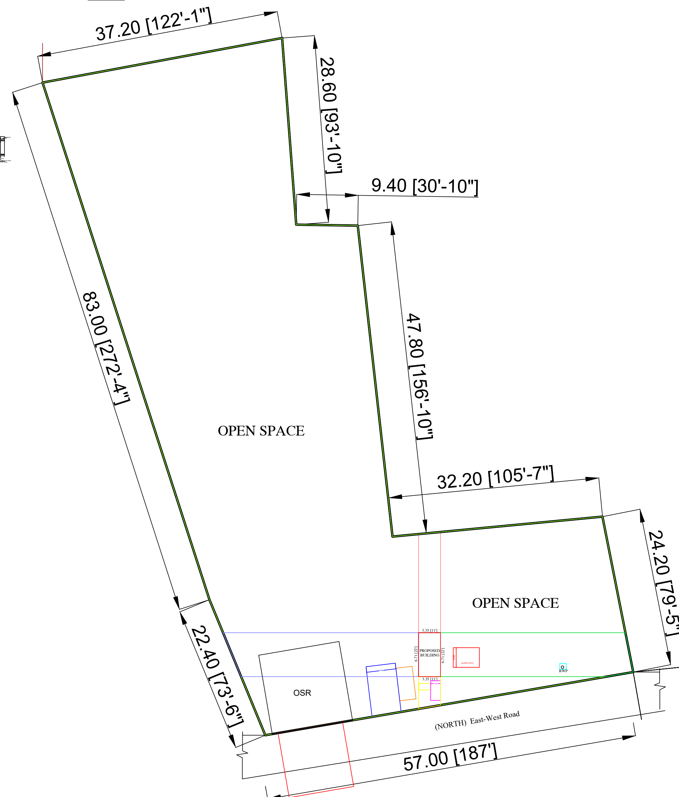
SITE PLAN-1
