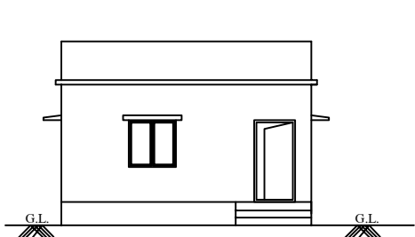
ELEVATION
