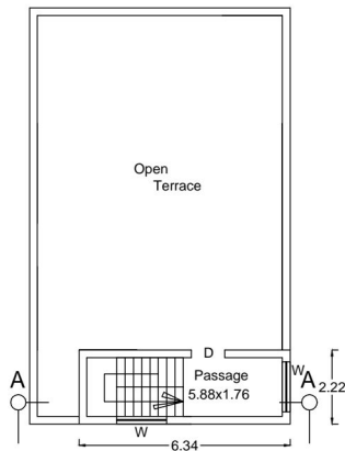
PLAN - F.F
