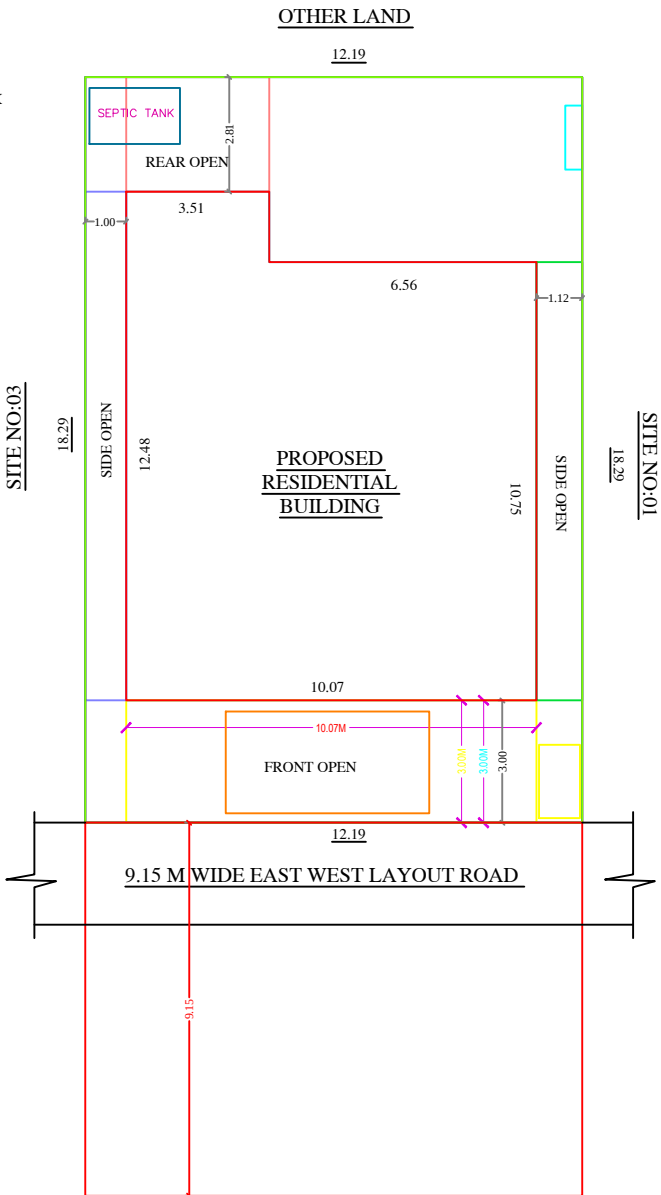
SITE PLAN 1:100
