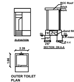
OUTER TOILET PLAN
