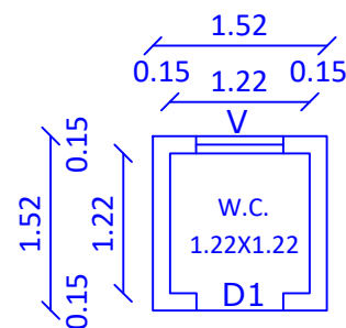
TOILET PLAN
