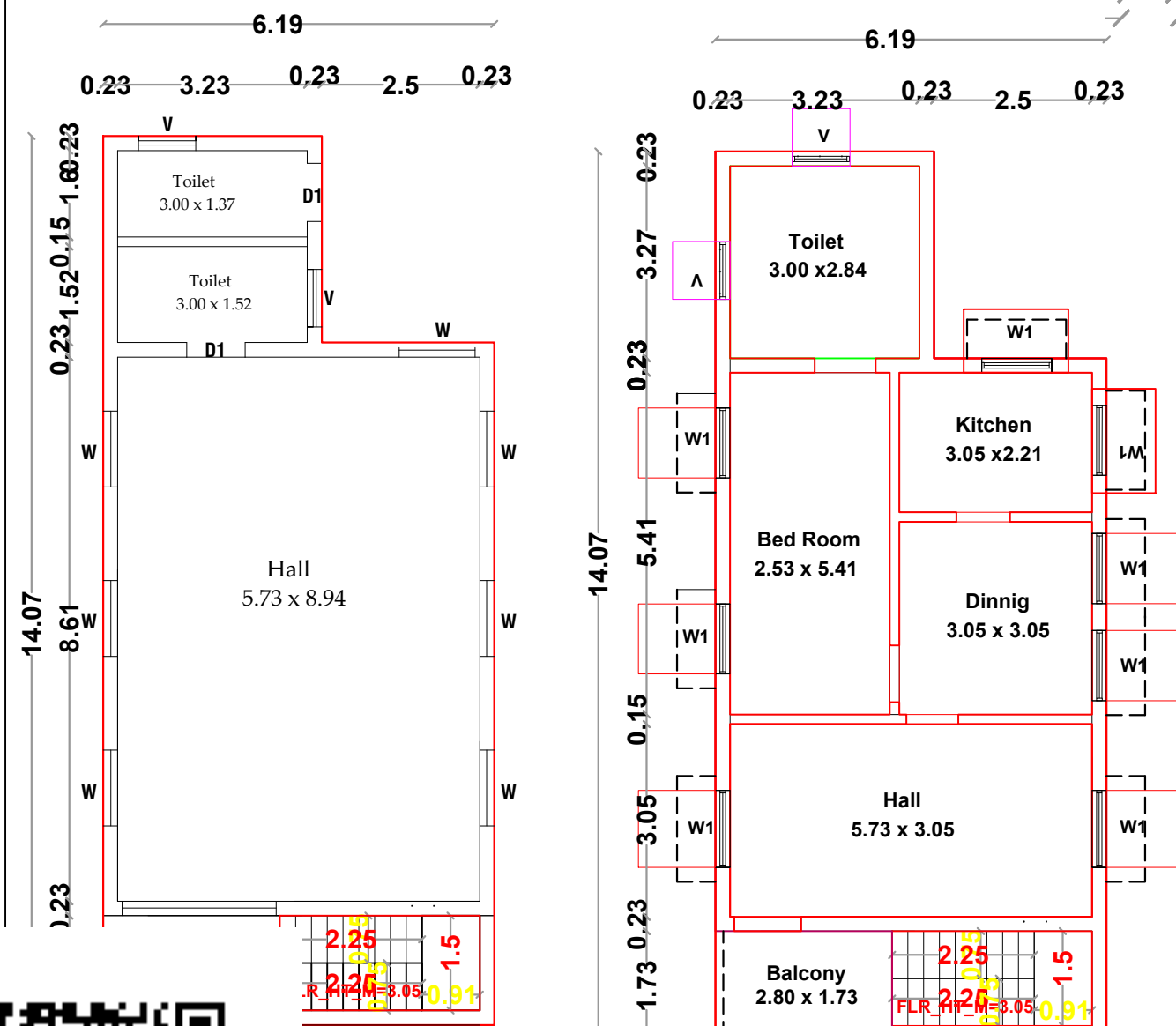
PRO. ADDI. FIRST FLOOR PLAN
