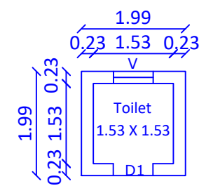
TOILET PLAN
