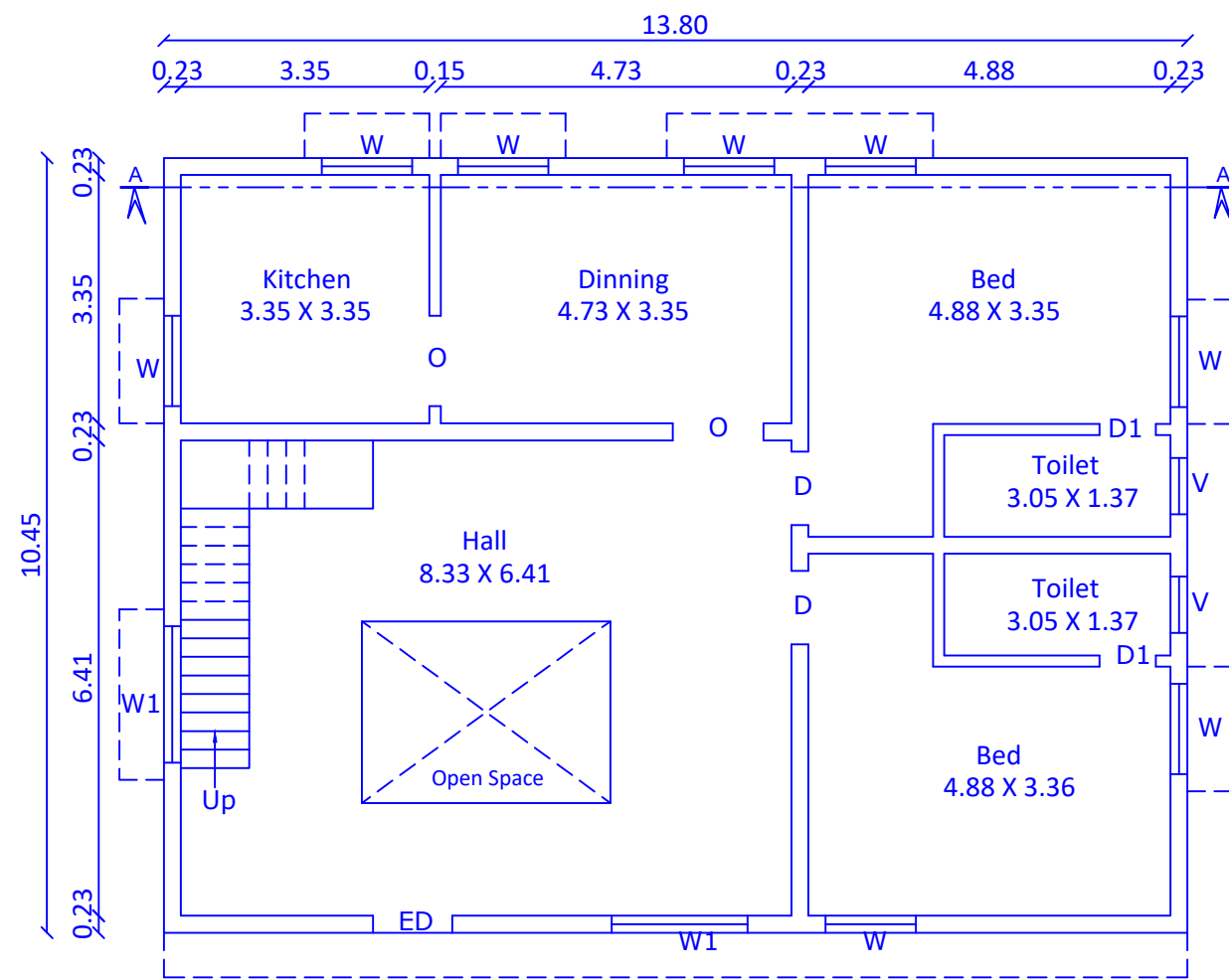
DOOR PLAN
