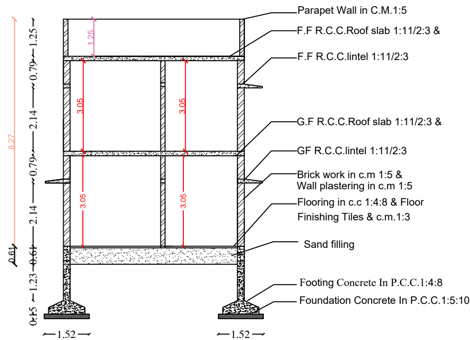
SECTION ON AB & A'B'
