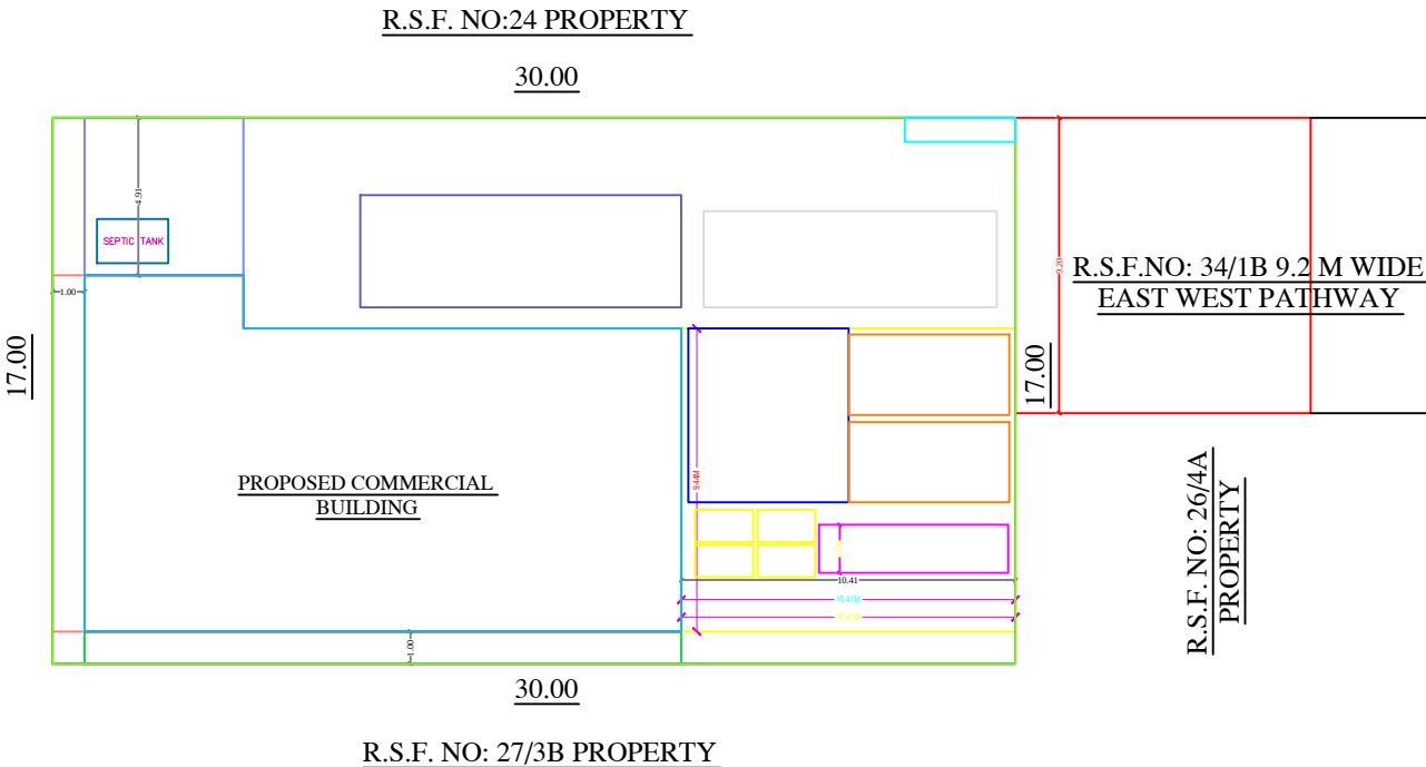
SITE PLAN 1:100
