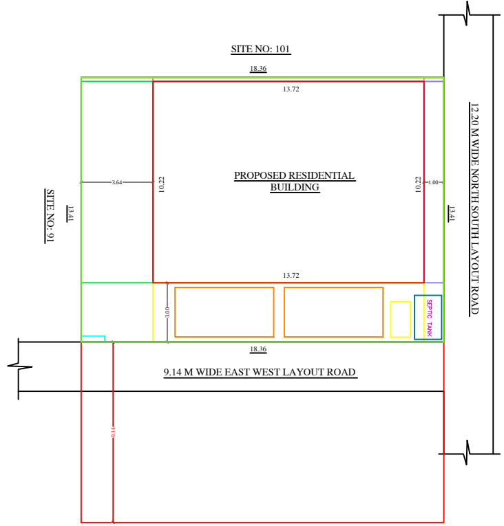
SITE PLAN 1:100
