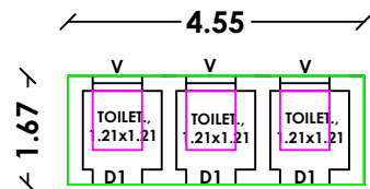
TOILET PLAN
