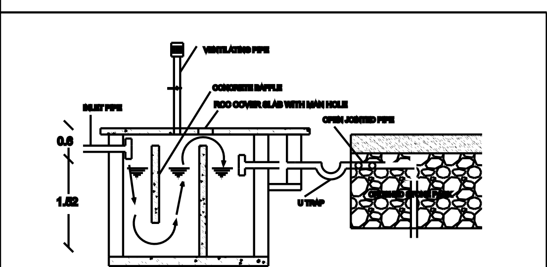
LONGITUDINAL SECTION
