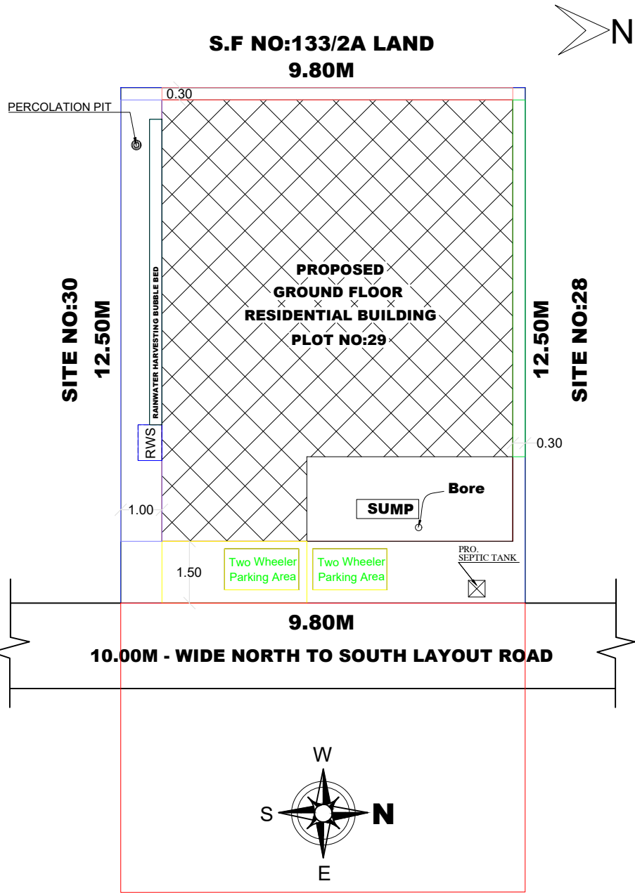
SITE PLAN (SCALE: 1:1)
