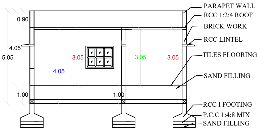
SECTION A-B
