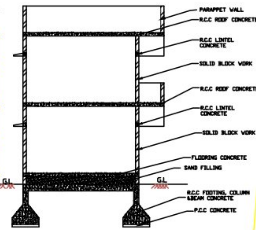
SECTION - A-B
