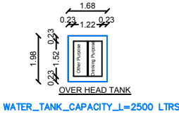
WATER_TANK_CAPACITY_L=2500 LTRS
