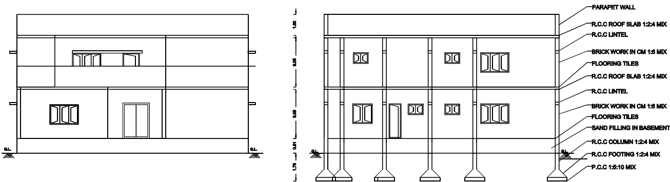
ELEVATION
