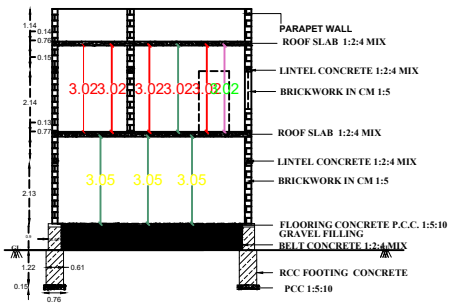
SECTION AA&A'
