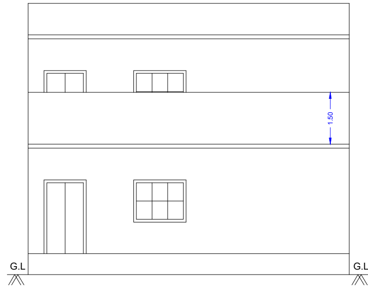
ELEVATION
