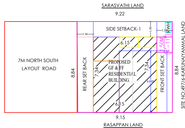
SITE PLAN 1:100
