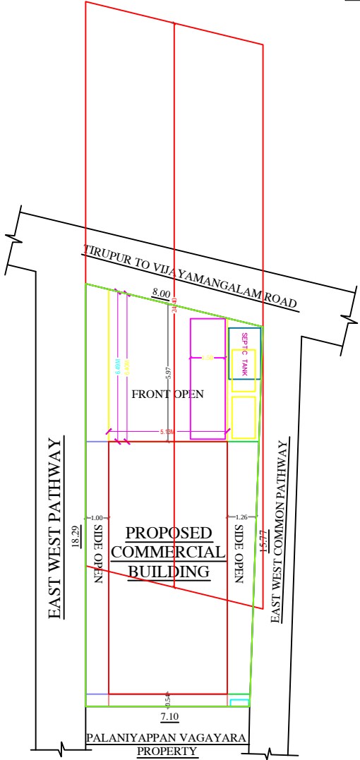
SITE PLAN 1:100
