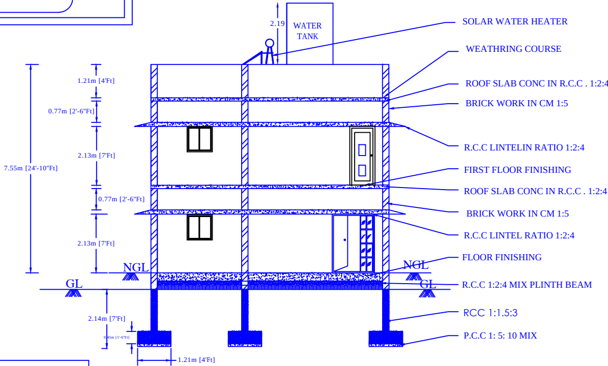
SECTION A-AA
