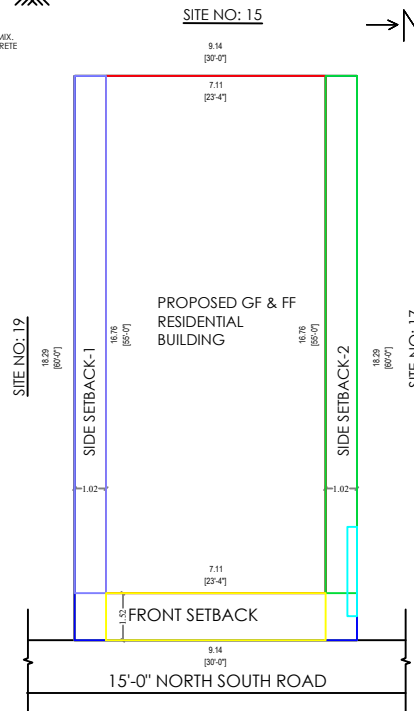
SITE PLAN 1:100
