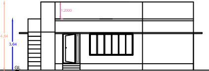
ELEVATION
