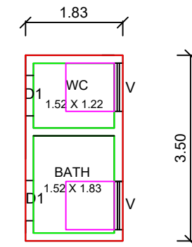
OUTER TOILET PLAN
