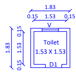
TOILET PLAN
