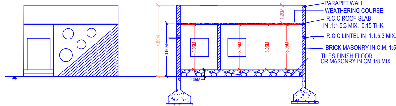
ELEVATION
