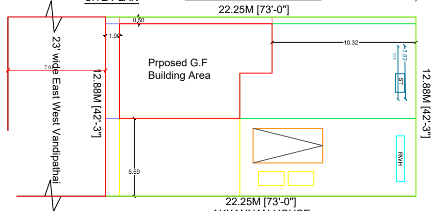
THANGAVEL AASARI LAND
