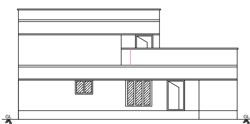
ELEVATION
