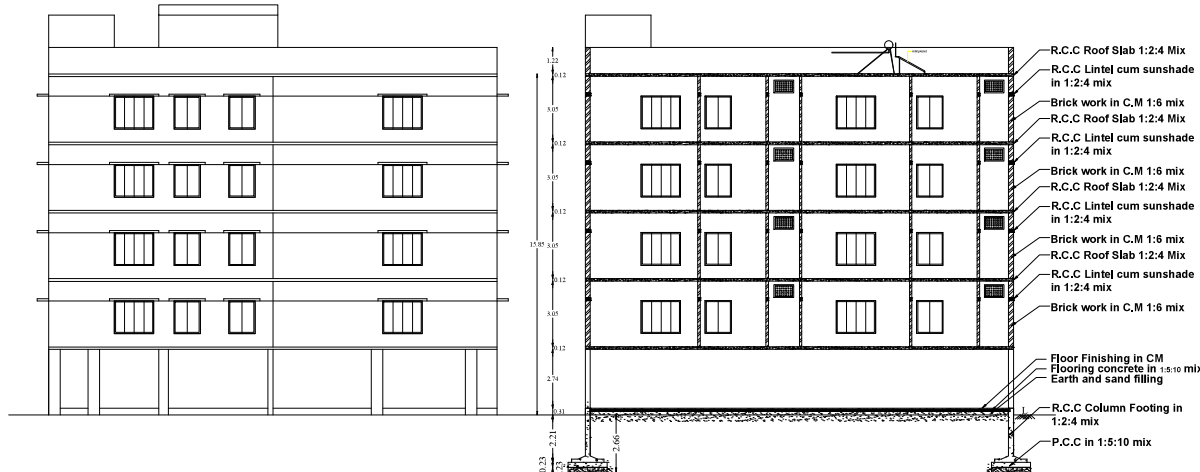
ELEVATION
