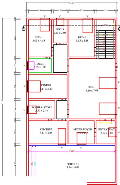
G.F.
