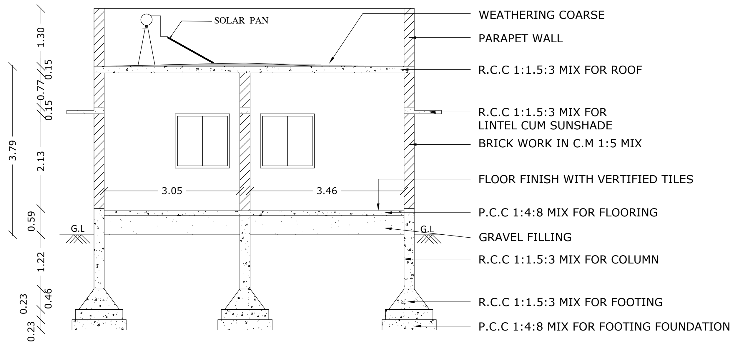
SECTION A-A'
