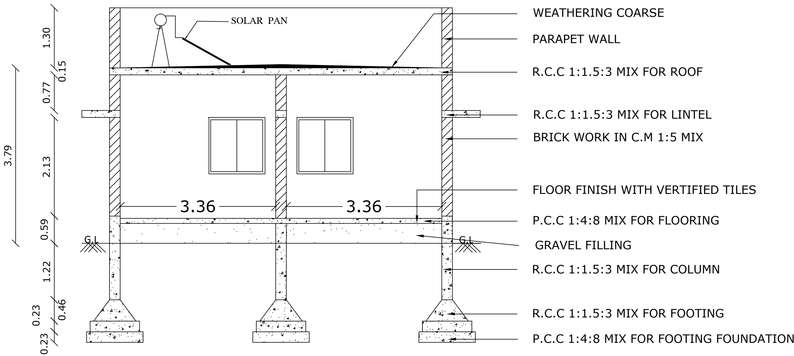
SECTION A-A'
