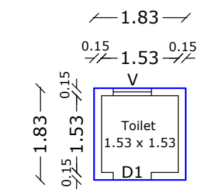
TOILET PLAN
