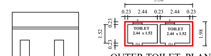
OUTER TOILET PLAN
