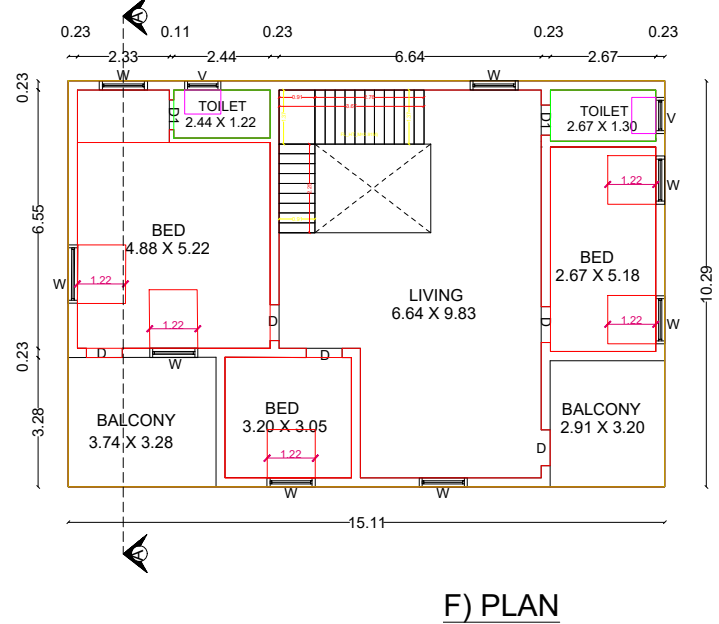
F) PLAN
