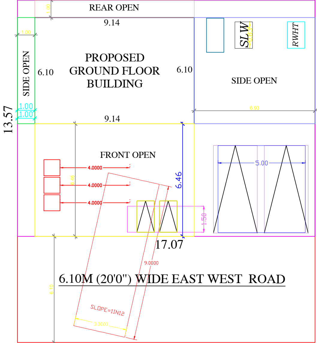
SITE PLAN 1:100
