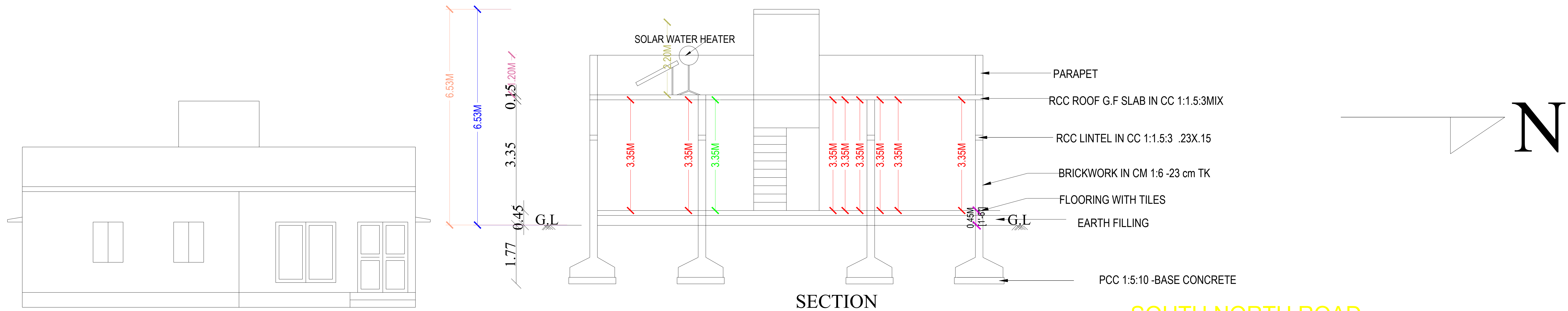
ELEVATION
