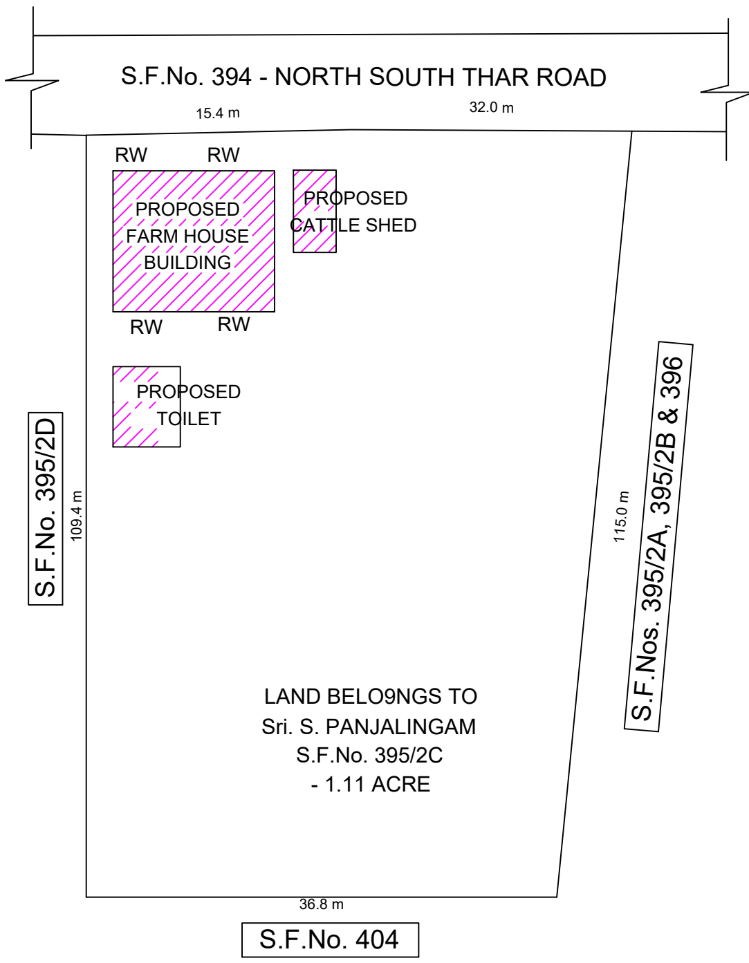
SITE PLAN SCALE : - NTS
