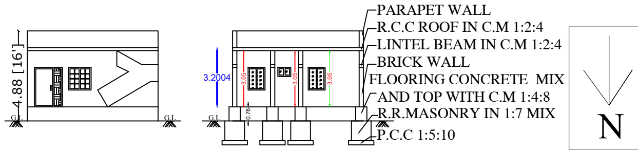
ELEVATION
