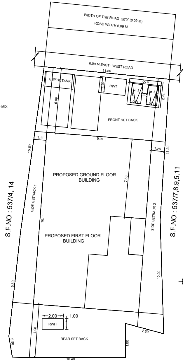
S.F.NO : 537/12 SITE PLAN
