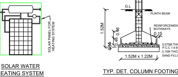
TYP. DET. COLUMN FOOTING
